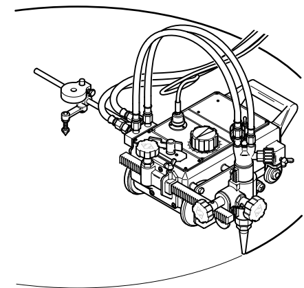
Découpage en chanfrein en V (avec deux chalumeaux)
